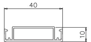
[中棧(テラス用)] 103-H
