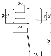
[ポール立用ブラケット] 220-H
