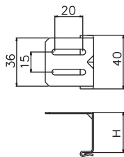
[カチコミ金具] 215□-H
