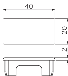
[中間金具] 213-H
