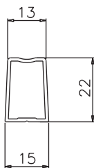
[横付金具] 212-H
