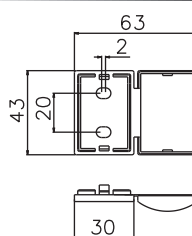
[化粧キャップ] 30
