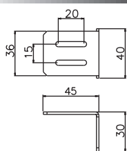
[横付金具] 212-H
