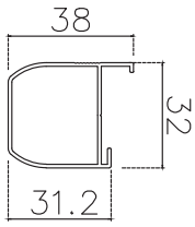
[縦框] 921-H
