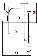
振止 148-H
