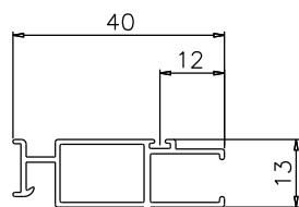
縦材 101-H
