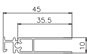
横材 102-H
