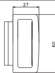
引手 127-H
